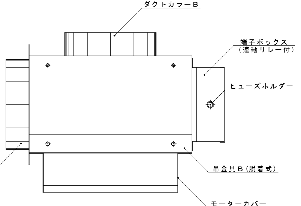
上面側
