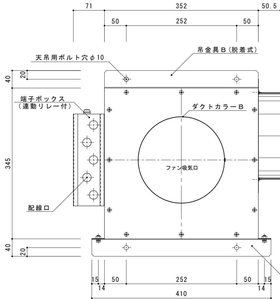
吸气側
