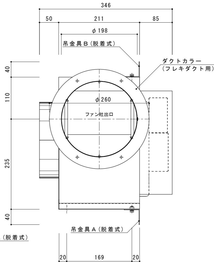
吐出側
